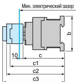
LC1 D09...D18 (3 полюса)
